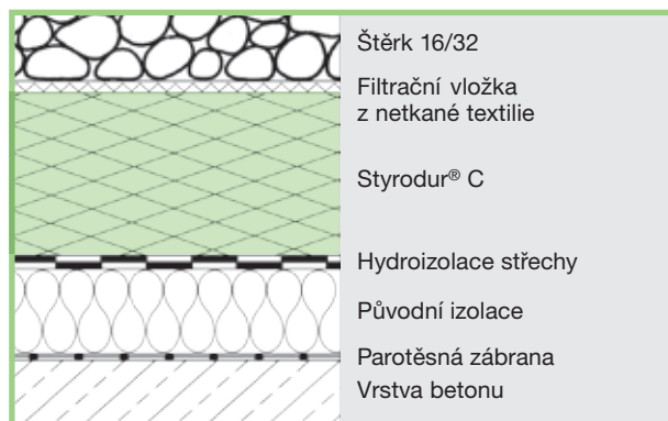
Obr. 3: Duo střecha s materiálem Styrodur C.
