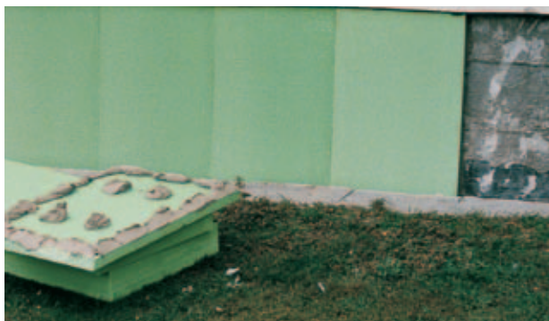
Obr. 14: Sanace staré stavby: Nalepení desek Styrodur® 2800 C bodově.
