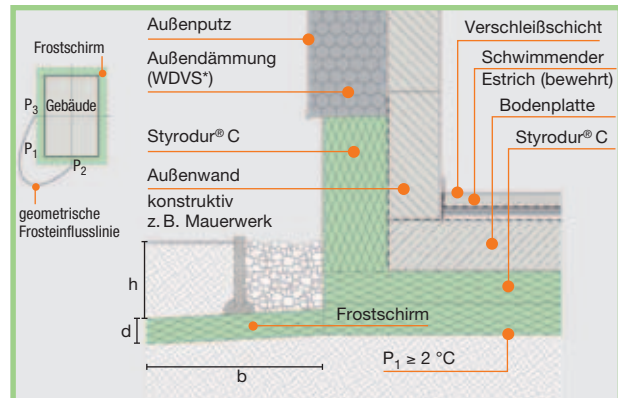
Abb. 5: Hinweis zur Ausführung eines Frostschirms.
